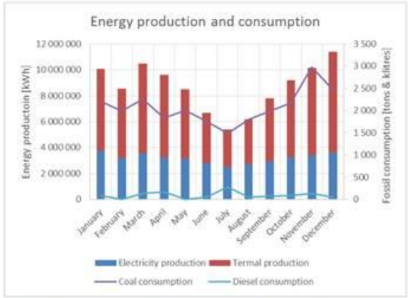
Figur 2 Månedlig energiproduksjon (søyler) og fossilt energiforbruk (linjer) for Longyearbyen energisentral i 2014.
