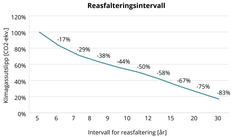
Figur 8: Mulige reduksjoner i klimagassutslipp for ulike intervaller for reasfaltering i løpet av en periode på 60 år. Tallene over grafen indikerer prosentvis reduksjon sammenlignet med reasfaltering hvert 5. år.
